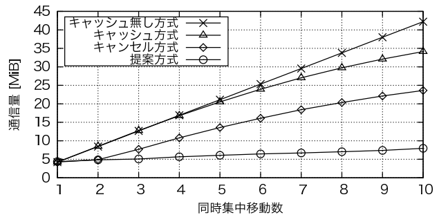
図 1 同時集中移動数に対する通信量の変化
