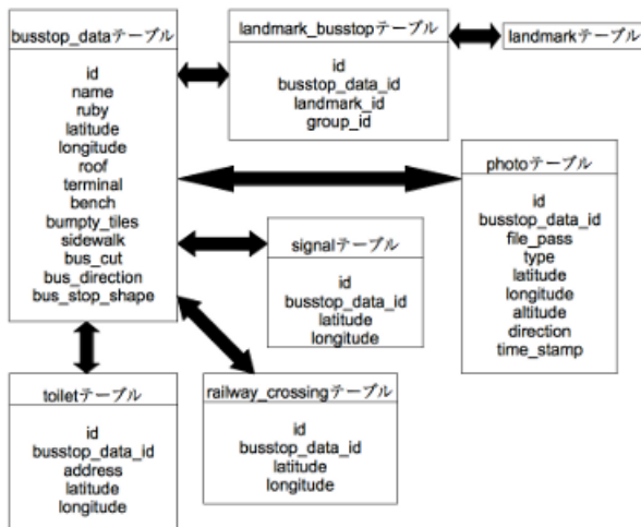
図7: 受け渡しのためのデータベース構造
