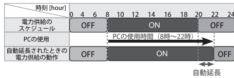
図 9 電力供給の延長動作例
