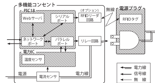
図2 多機能コンセントの構成 Fig.2 Configuration of the multifunctional electrical outlet.
